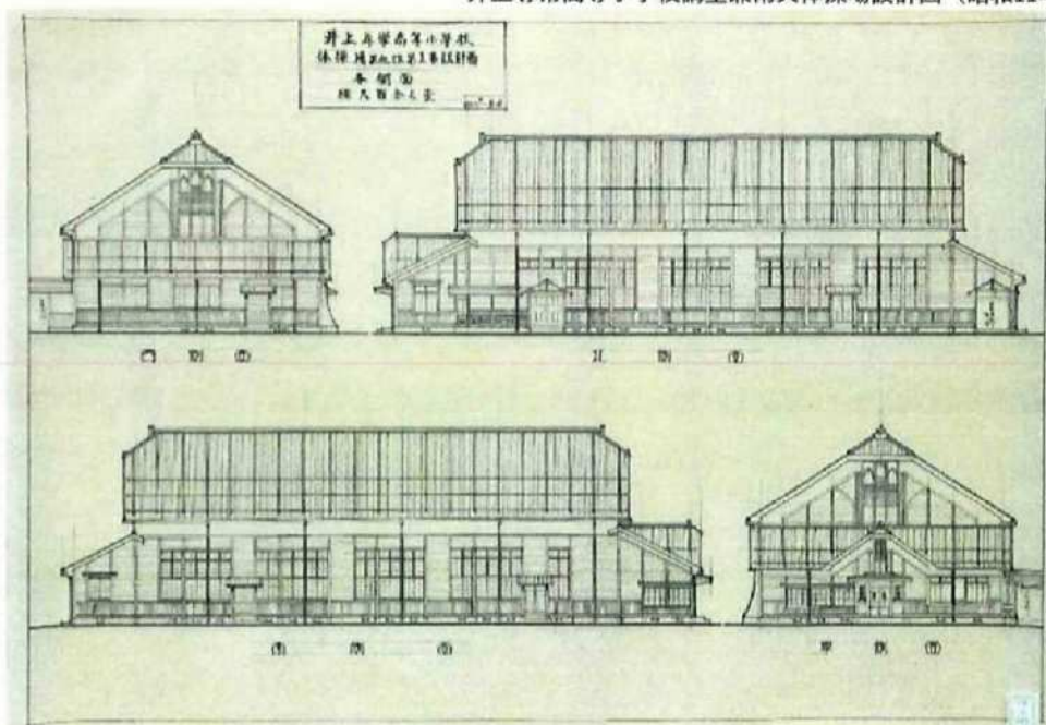
井上尋常高等小学校講堂兼雨天体操場設計図（昭和11年）
