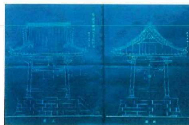
広円寺鐘樓改築工事設計図（昭和12年）
