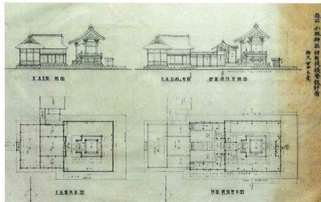
縣社小坂神社移転模様替設計図（昭和16年）
