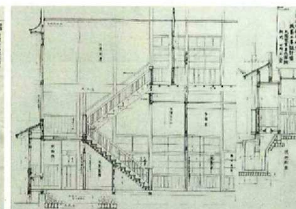
須坂町庁舎改築工事設計図 北階段室其他詳細（昭和13年）
